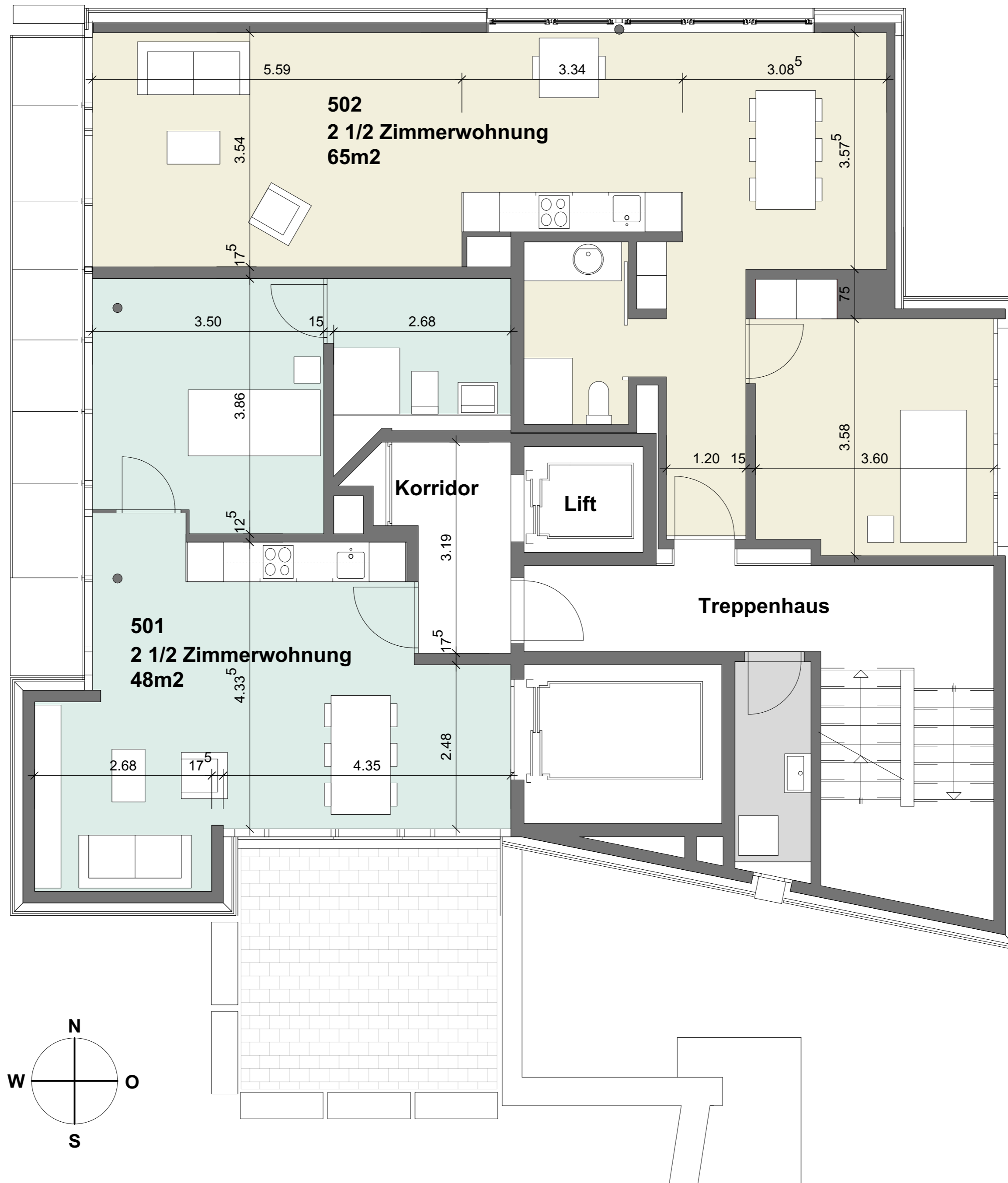
Lindenpark Windisch - Wohnungen 5. Obergeschoss
